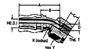
45° elbow bent tube
